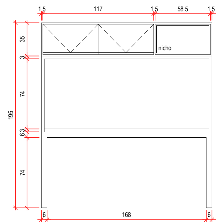
VISTA FRONTAL | mesa + armário aéreo ESC 1/25
