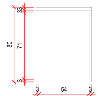
VISTA LATERAL | aparador ESC 1/25
