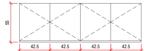
VISTA FRONTAL | armário aéreo pia cozinha ESC 1/25
