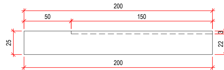
VISTA SUPERIOR | painel tv ESC 1/25
