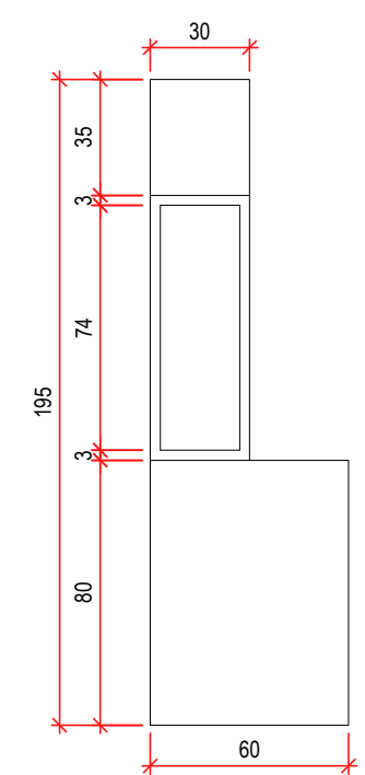
VISTA LATERAL | mesa ESC 1/25
