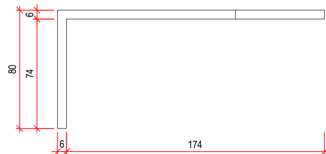
VISTA FRONTAL | mesa ESC 1/25
