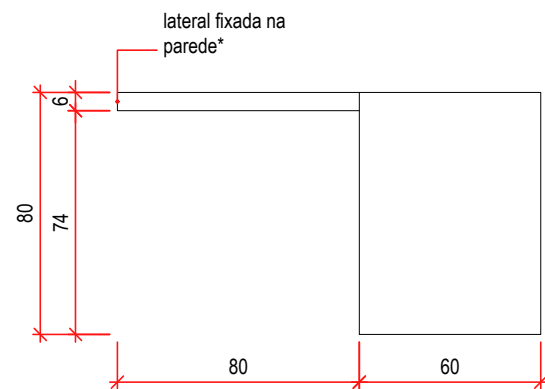
VISTA LATERAL | mesa ESC 1/25
